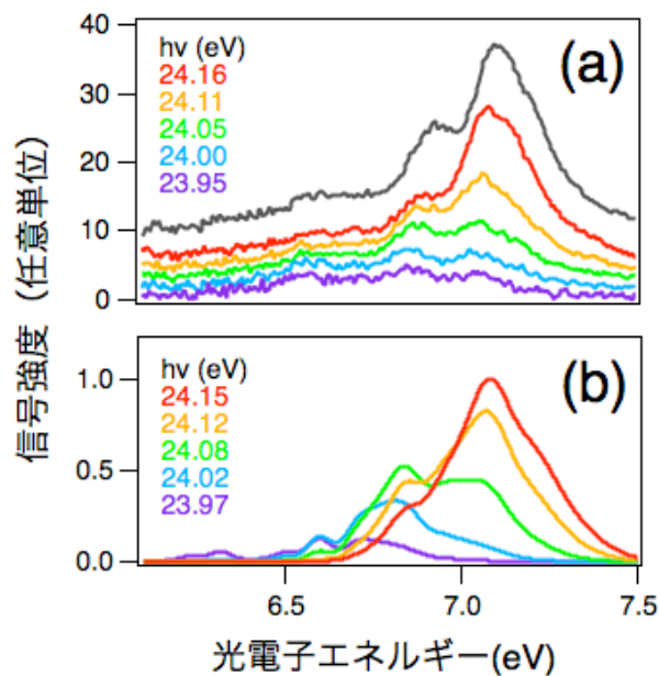
図 2 : ピーク (A) の拡大図。いくつかの小さいピークが見られる (黒線)。光の「ゆらぎ」を利用した実験計測 (a) と理論計算 (b) からこれらのサブピークは 2 電子励起状態に由来することがわかる。
