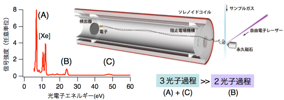
図 1 : 光電子エネルギーの計測に用いた磁気ボトル型光電子分光器 (右) とヘリウムに極紫外 (波長 51 nm) 強レーザーパルス照射したときの光電子エネルギースペクトル (左)
